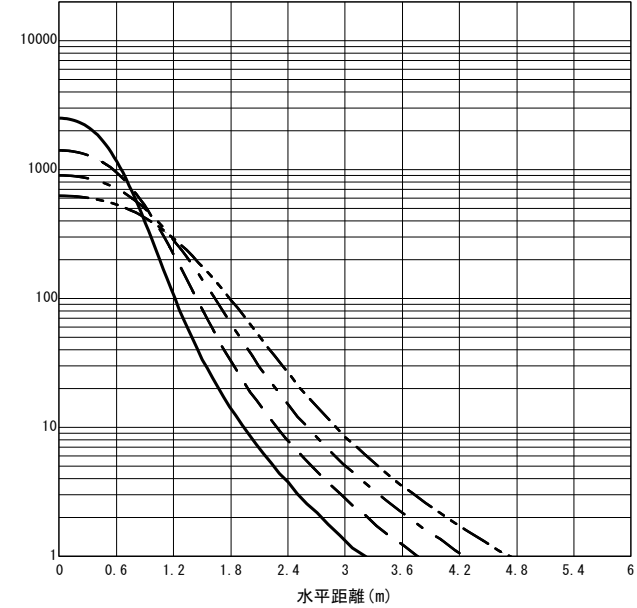
○直射水平面照度 (全光束: 3780 × 1 = 3780lm/台) 照度 (lx) — H1.50m --- H2.00m - - - H2.50m - · - · H3.00m (保守率: 1.00)
