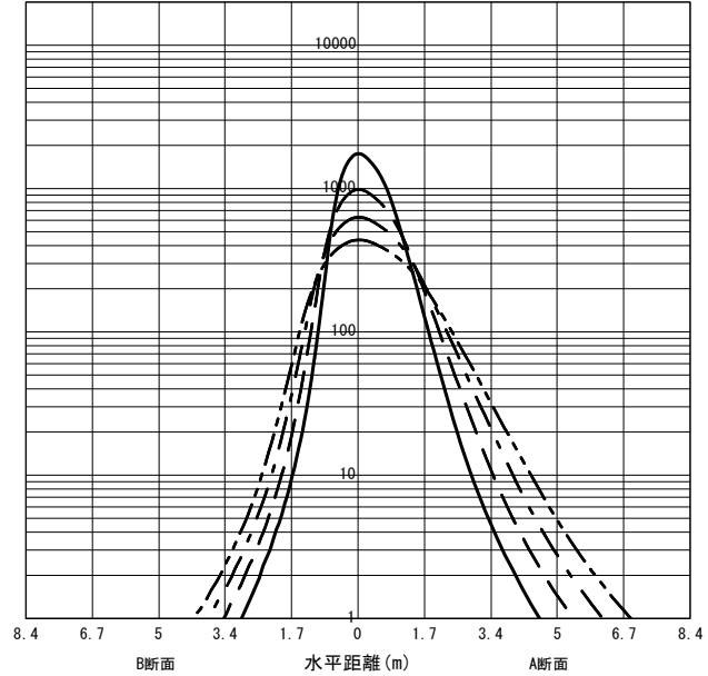
○直射水平面照度 (全光束: 3840 × 1 = 3840lm/台) 照度 (lx) — H1.50m --- H2.00m - - - H2.50m - · - · H3.00m (保守率: 1.00)
