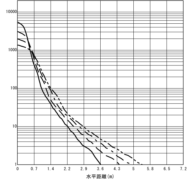
○直射水平面照度 (全光束: 3940 × 1 = 3940lm/台) 照度 (lx) — H1.50m --- H2.00m - - - H2.50m - · - · H3.00m (保守率: 1.00)
