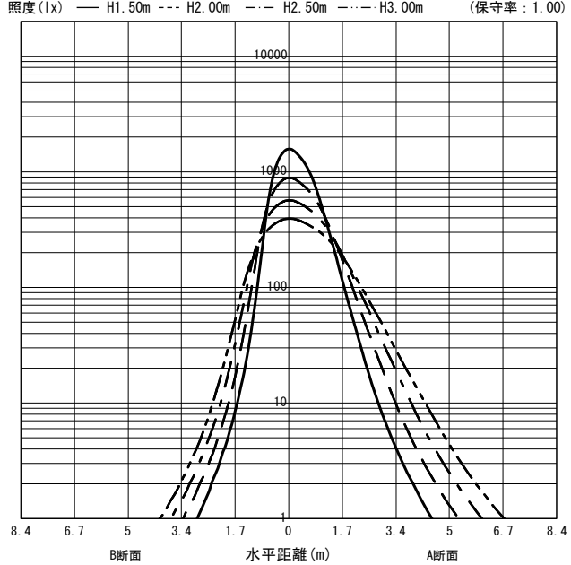
○直射水平面照度 (全光束 : 3455 × 1 = 3455lm/台)
