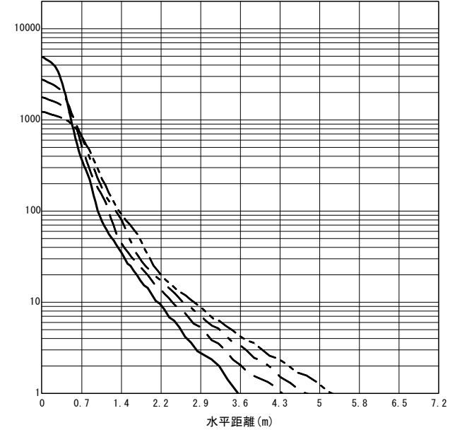
○直射水平面照度 (全光束 : 3545 × 1 = 3545lm/台) 照度 (lx) — H1.50m --- H2.00m - - - H2.50m - · - · H3.00m (保守率 : 1.00)
