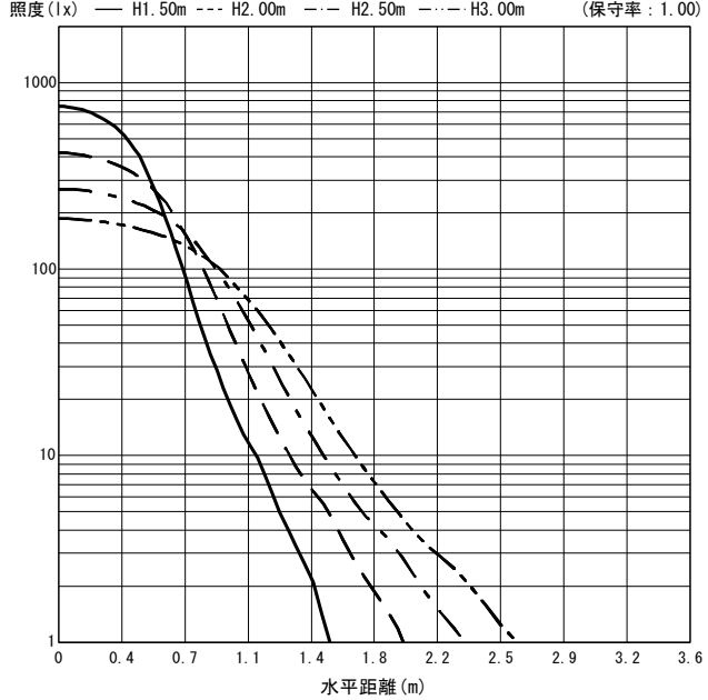
○直射水平面照度 (全光束 : 680 × 1 = 680lm/台)
