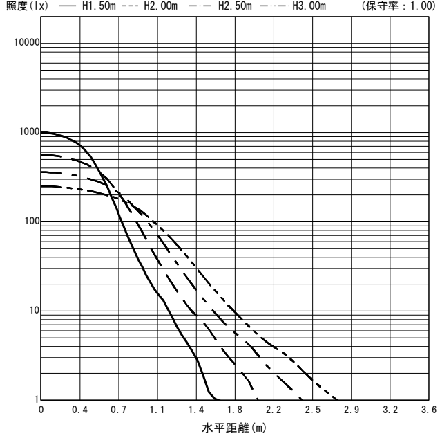
○直射水平面照度 (全光束: 910 × 1 = 910lm/台)
