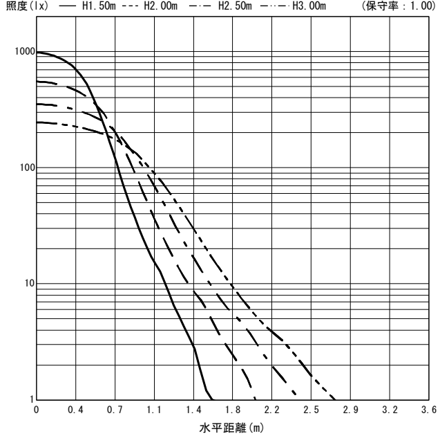
○直射水平面照度 (全光束: 890 × 1 = 890lm/台)
