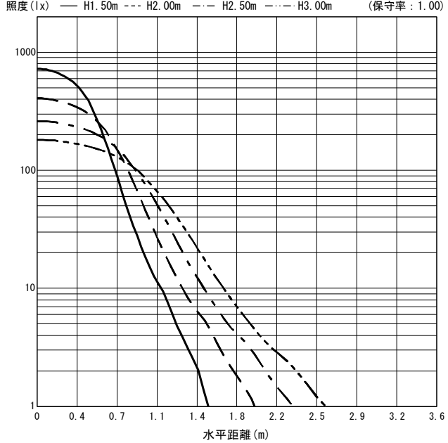
○直射水平面照度 (全光束 : 660 × 1 = 660lm/台)
