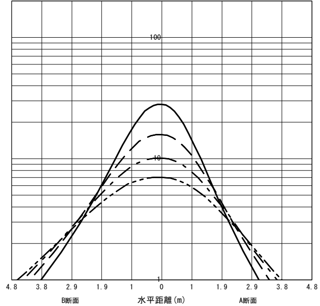
○直射水平面照度 (全光束 : 360 × 1 = 360lm/台) 照度 (lx) — H1.50m --- H2.00m - - - H2.50m - · - · H3.00m (保守率 : 1.00)
