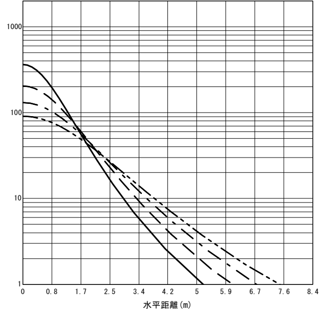
○直射水平面照度 (全光束: 1980 × 1 = 1980lm/台) 照度 (lx) — H1.50m --- H2.00m - - - H2.50m - · - · H3.00m (保守率: 1.00)
