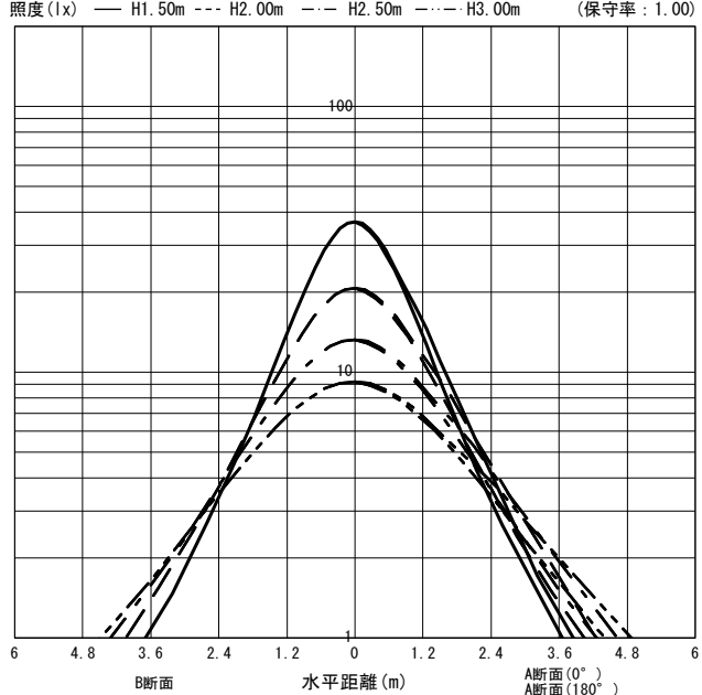
○直射性水平面照度 (全光束: 760 × 1 = 760lm/台)
