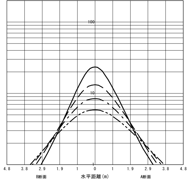
○直射水平面照度 (全光束: 560 × 1 = 560lm/台) 照度 (lx) — H1.50m --- H2.00m - - - H2.50m - · - · H3.00m (保守率: 1.00)
