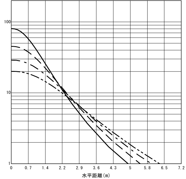
○直射水平面照度 (全光束: 1030 × 1 = 1030lm/台) 照度 (lx) — H1.50m --- H2.00m - - - H2.50m - · - · H3.00m (保守率: 1.00)
