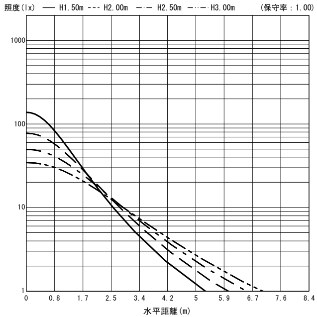
○直射水平面照度 (全光束: 1380 × 1 = 1380lm/台)
