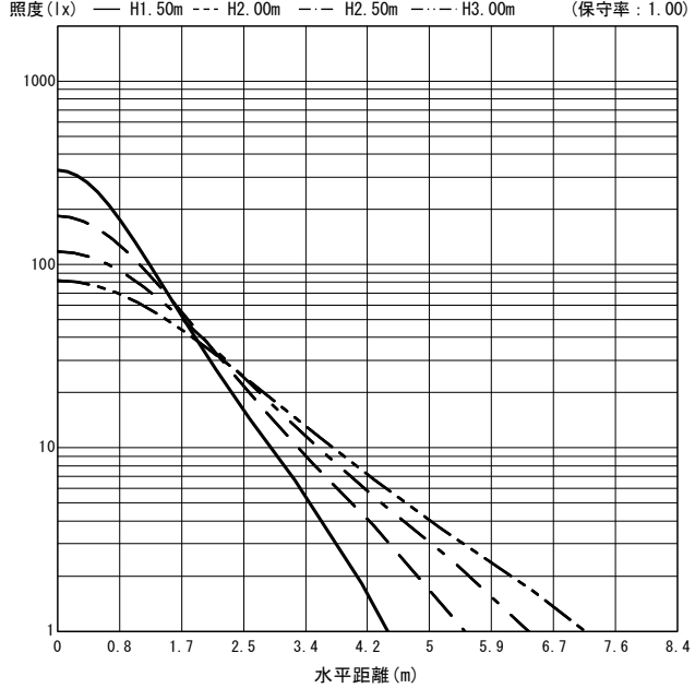
○直射水平面照度 (全光束: 1750 × 1 = 1750lm/台)
