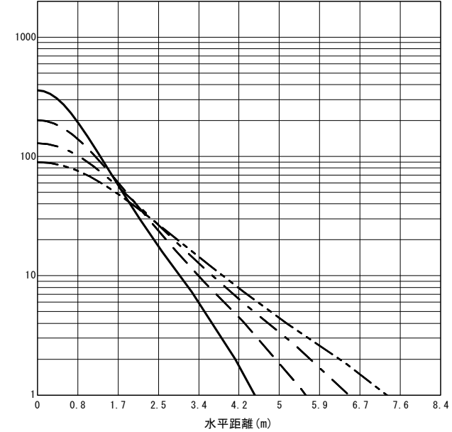
○直射水平面照度 (全光束: 1920 × 1 = 1920lm/台) 照度 (lx) — H1.50m --- H2.00m - - - H2.50m - · - · H3.00m (保守率: 1.00)
