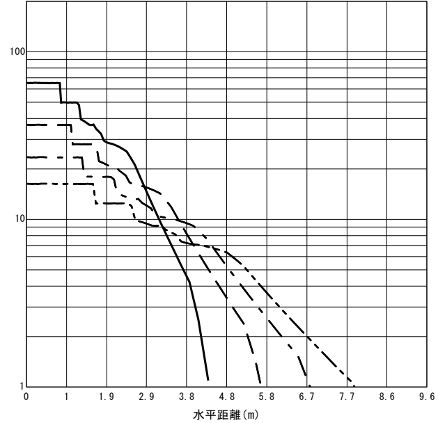
○直射水平面照度 (全光束: 1055 × 1 = 1055lm/台) 照度 (lx) — H1.50m --- H2.00m - - - H2.50m - · - · H3.00m (保守率: 1.00)
