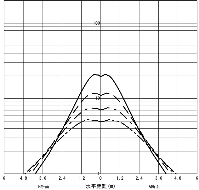
○直射水平面照度 (全光束 : 920 × 1 = 920lm/台) 照度 (lx) — H1.50m --- H2.00m - - - H2.50m - · - · H3.00m (保守率 : 1.00)
