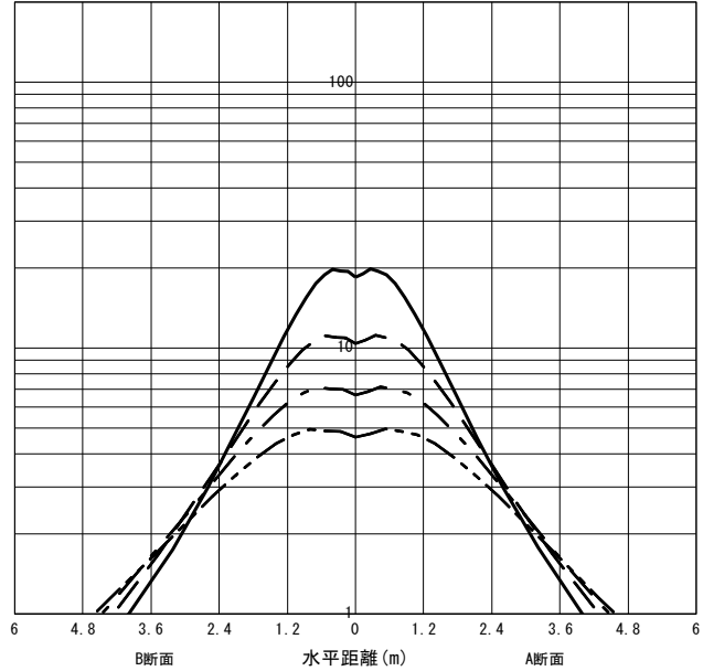
○直射水平面照度 (全光束 : 870 × 1 = 870lm/台) 照度 (lx) — H1.50m --- H2.00m - - - H2.50m - · - · H3.00m (保守率 : 1.00)
