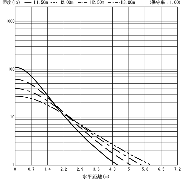
○直射水平面照度 (全光束 : 760 × 2 = 1520lm/台)
