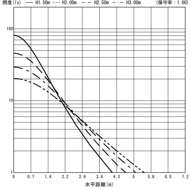
○直射水平面照度 (全光束 : 560 × 2 = 1120lm/台)
