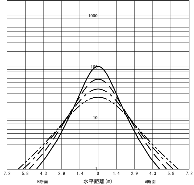
○直射水平面照度 (全光束 : 760 × 3 = 2280lm/台)
