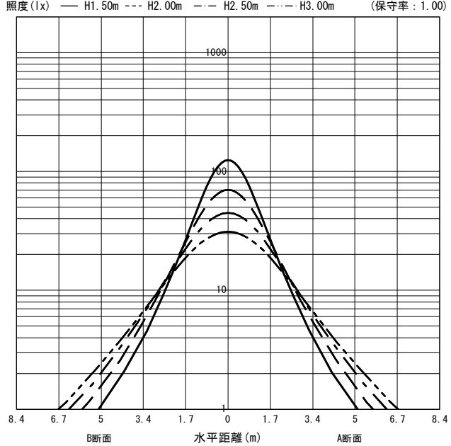
○直射水平面照度 (全光束 : 920 × 3 = 2760lm/台)
