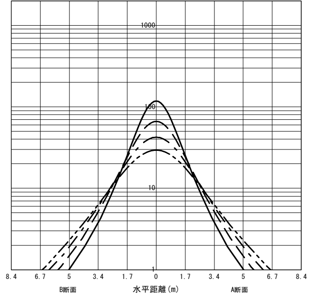
○直射水平面照度 (全光束 : 870 × 3 = 2610lm/台) 照度 (lx) — H1.50m --- H2.00m - - - H2.50m - · - · H3.00m (保守率 : 1.00)
