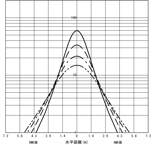
○直射水平面照度 (全光束 : 440 × 3 = 1320lm/台) 照度 (lx) — H1.50m --- H2.00m - - - H2.50m - · - · H3.00m (保守率 : 1.00)
