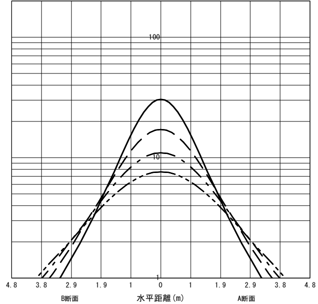
○直射水平面照度 (全光束: 410 × 1 = 410lm/台) 照度 (lx) — H1.50m --- H2.00m - - - H2.50m - · - · H3.00m (保守率: 1.00)
