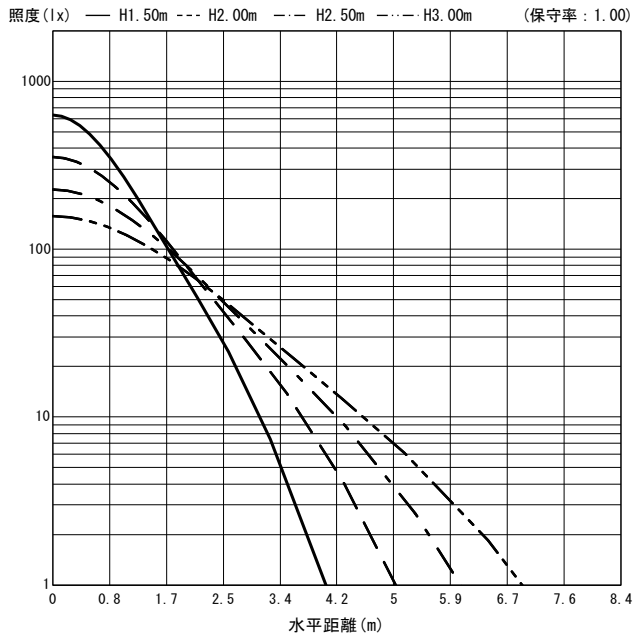
○直射水平面照度 (全光束: 3240 × 1 = 3240lm/台)
