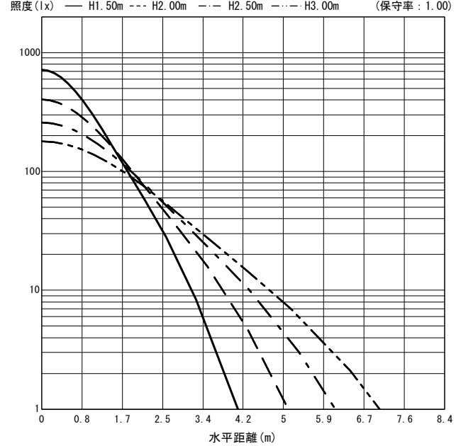
○直射水平面照度 (全光束: 3690 × 1 = 3690lm/台)
