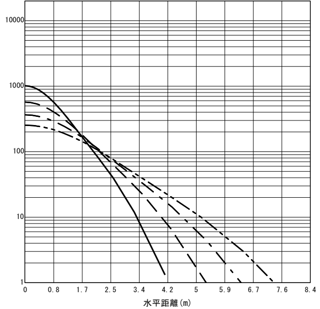
○直射水平面照度 (全光束: 5210 × 1 = 5210lm/台)
