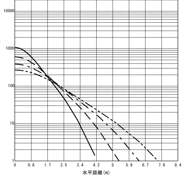
○直射水平面照度 (全光束: 5530 × 1 = 5530lm/台) 照度 (lx) — H1.50m --- H2.00m - - - H2.50m - · - · H3.00m (保守率: 1.00)
