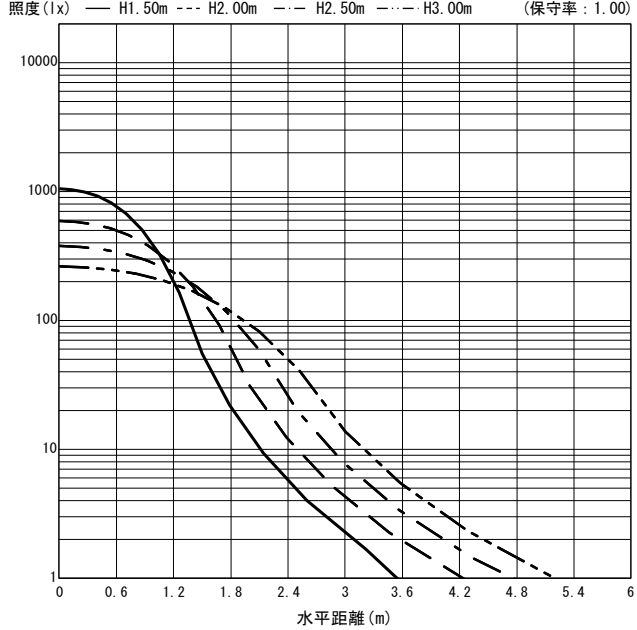
○直射水平面照度 (全光束 : 3090 × 1 = 3090lm/台)
