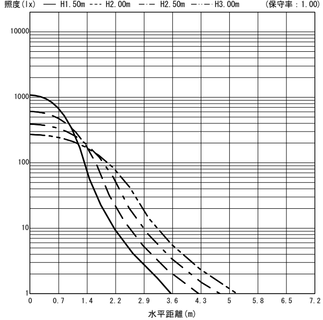
○直射水平面照度 (全光束 : 3180 × 1 = 3180lm/台)
