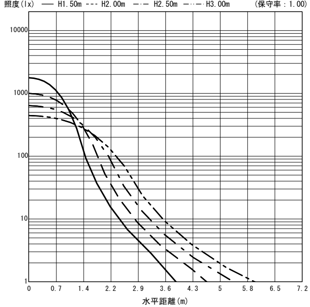
○直射水平面照度 (全光束: 5210 × 1 = 5210lm/台)
