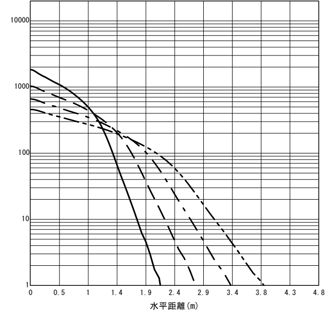
○直射水平面照度 (全光束: 3560 × 1 = 3560lm/台) 照度 (lx) — H1.50m --- H2.00m - - - H2.50m - · - · H3.00m (保守率: 1.00)
