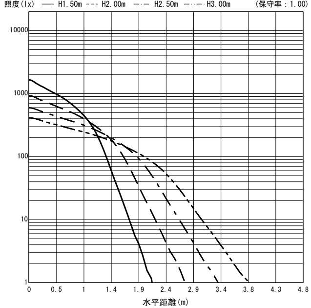
○直射水平面照度 (全光束 : 3220 × 1 = 3220lm/台)
