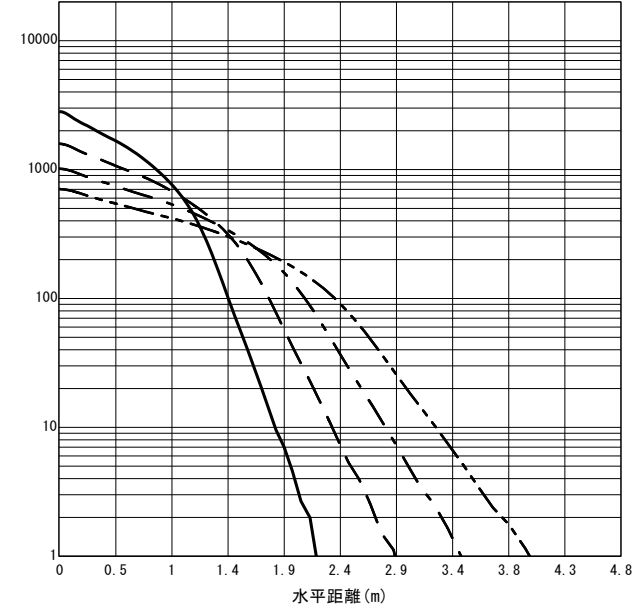
○直射水平面照度 (全光束 : 5480 × 1 = 5480lm/台) 照度 (lx) — H1.50m --- H2.00m - - - H2.50m - · - · H3.00m (保守率 : 1.00)
