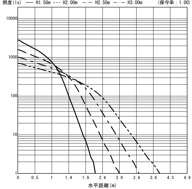
○直射水平面照度 (全光束: 5470 × 1 = 5470lm/台)
