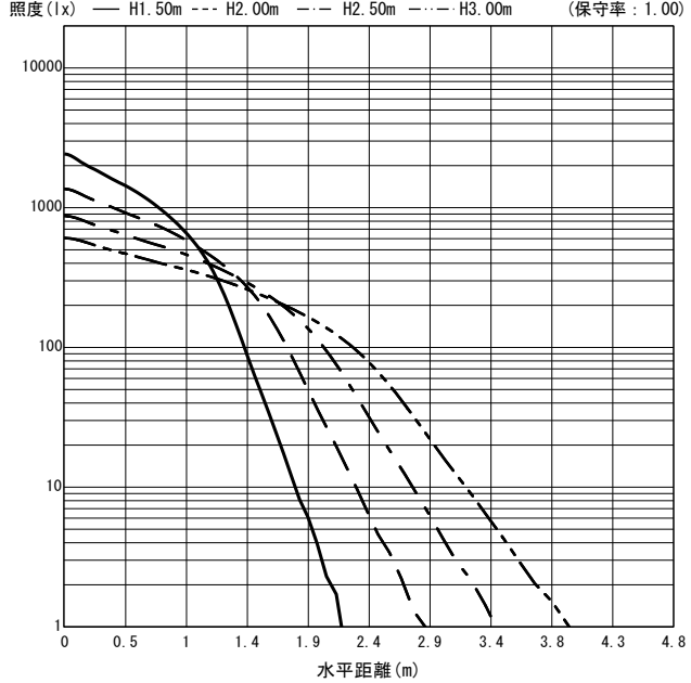
○直射水平面照度 (全光束 : 4710 × 1 = 4710lm/台)
