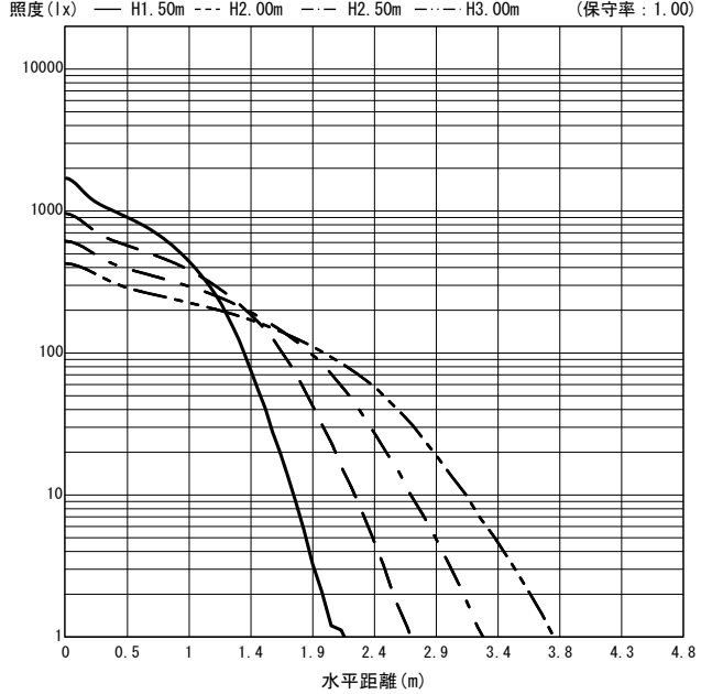
○直射水平面照度 (全光束: 3150 × 1 = 3150lm/台)
