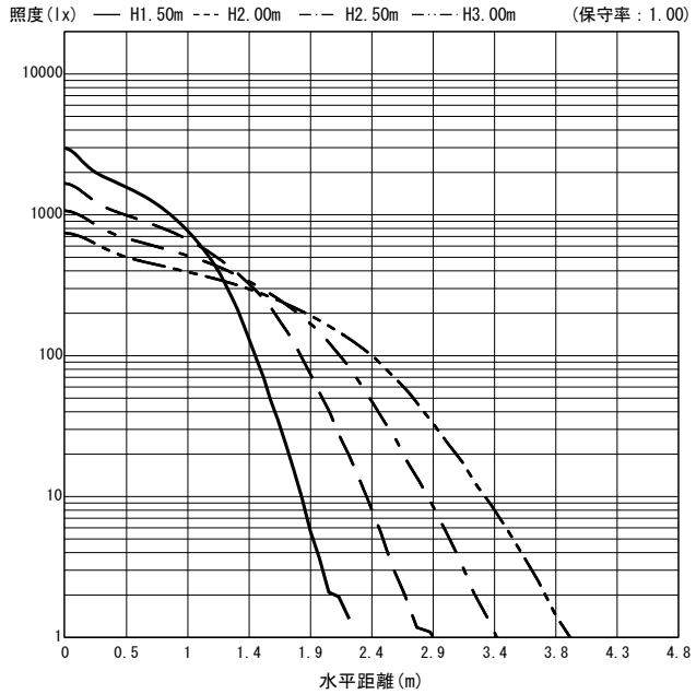
○直射水平面照度 (全光束: 5480 × 1 = 5480lm/台)
