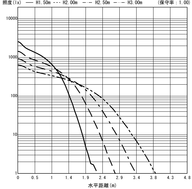
○直射水平面照度 (全光束 : 4720 × 1 = 4720lm/台)
