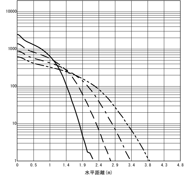
○直射水平面照度 (全光束: 4570 × 1 = 4570lm/台) 照度 (lx) — H1.50m --- H2.00m - - - H2.50m - · - · H3.00m (保守率: 1.00)
