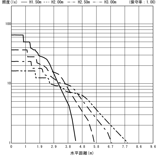
○直射水平面照度 (全光束: 1055 × 1 = 1055lm/台)
