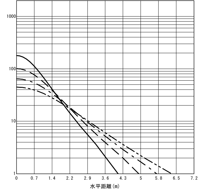
○直射水平面照度 (全光束: 960 × 1 = 960lm/台) 照度 (lx) — H1.50m --- H2.00m - - - H2.50m - · - · H3.00m (保守率: 1.00)
