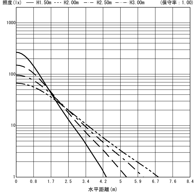
○直射水平面照度 (全光束: 1430 × 1 = 1430lm/台)
