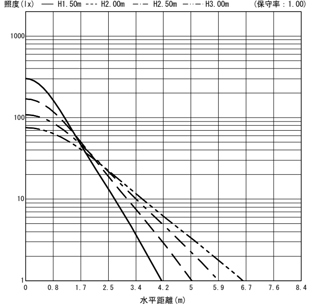
○直射水平面照度 (全光束: 1540 × 1 = 1540lm/台)
