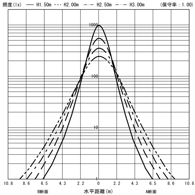
○直射水平面照度 (全光束: 3520 × 2 = 7040lm/台)
