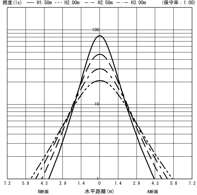
○直射水平面照度 (全光束: 550 × 1 = 550lm/台)
