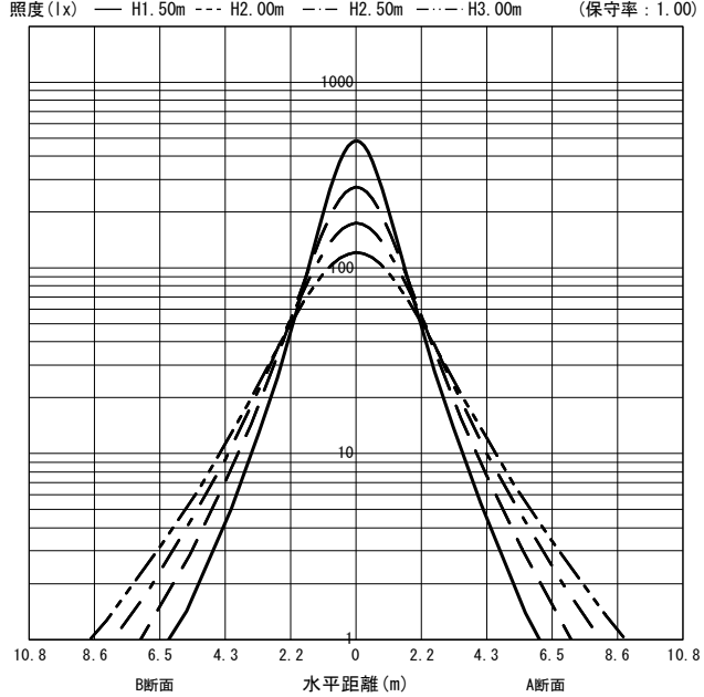
○直射水平面照度 (全光束: 3080 × 1 = 3080lm/台)
